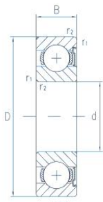
Z型 单侧带防尘盖
